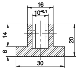
Presjek A-A
